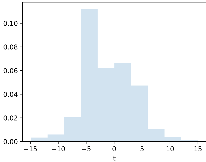
plt.hist(t, bins=10)
