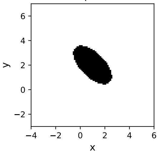
Ellipse2D
