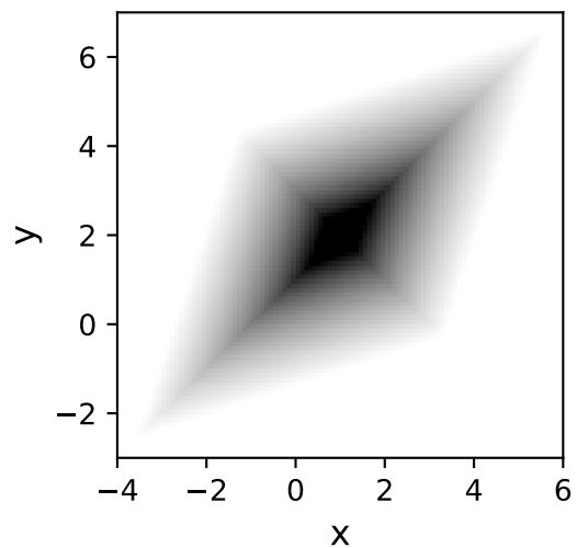
GeneralSersic2D, c=-1.0
